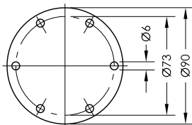
Flansch 85 nach DIN24557 Teil 2
